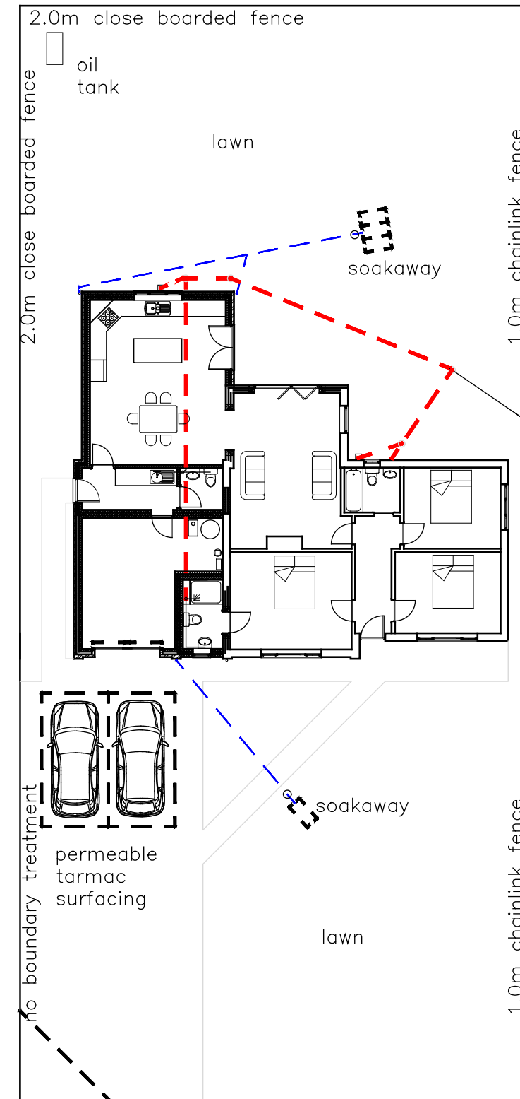
SITE LAYOUT 1.200
